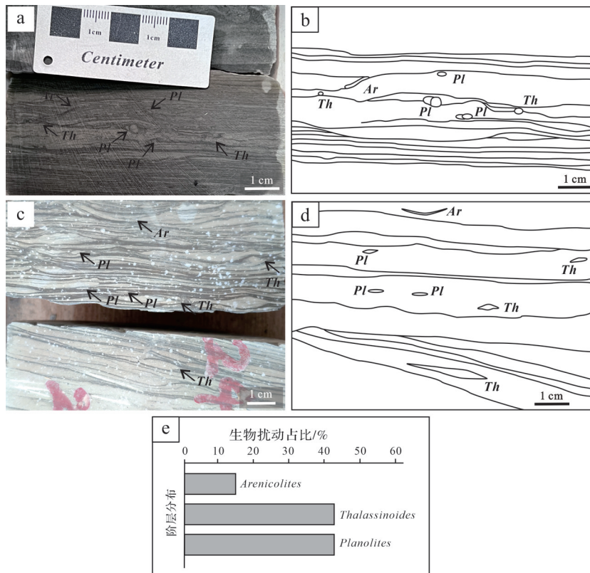
图5 Planolites 遗迹组
