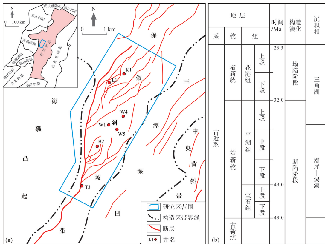
图1 西湖凹陷构造单元划分(a)及地层柱状图(b)(据屈童等,2024修改)
