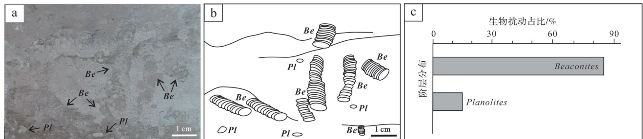
图8 Beaconites 遗迹组构
