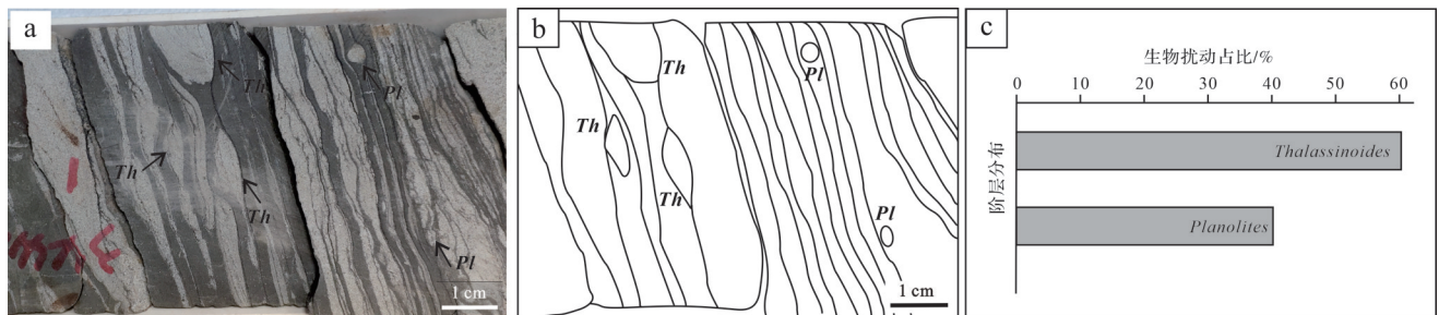
图6 Thalassinoides 遗迹组构
