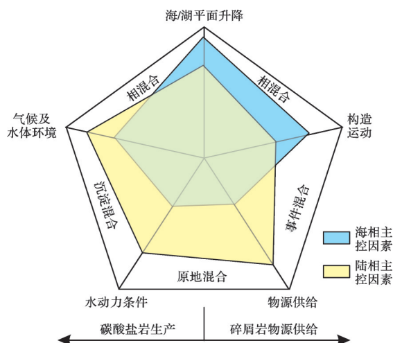
图8 混合沉积控制因素相互关系示意图
