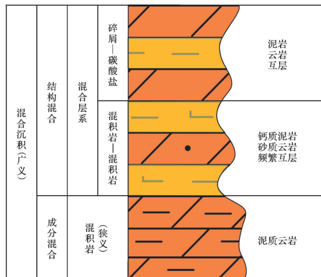
图 1 混合沉积类型与特征
