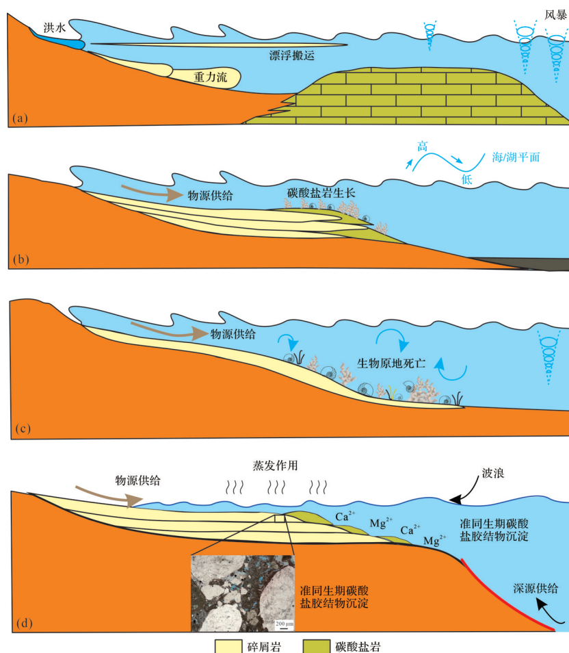
图6 混合沉积作用模式图
