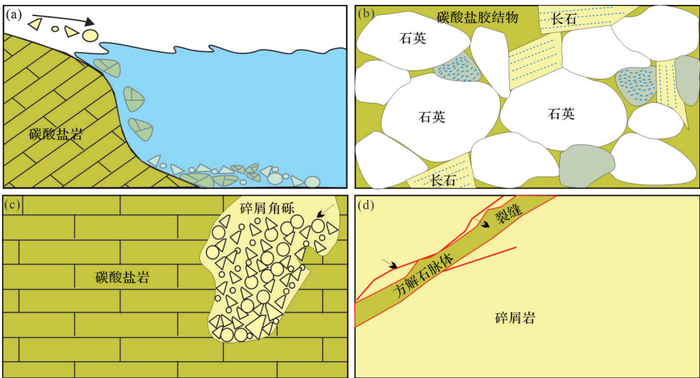
图7 假混合形成模式示意图 (a) 蚀源混合示意图: 碳酸盐岩经过搬运与碎屑岩一同沉积 [2] ; (b) 成岩混合示意图: 后期碳酸盐胶结物充填粒间孔, 胶结碎屑颗粒; (c) 岩溶混合: 碳酸盐岩发生岩溶作用, 后期碎屑颗粒充填溶洞 [20] ; (d) 裂缝混合: 碎屑岩中发育裂缝, 后期碳酸盐脉体充填裂缝 [20]
